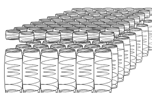
砂時計型ポケットコイル：【並列】 + 薄型インナーポケットコイル：【千鳥】
