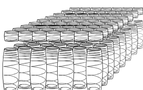
どんぐり型ポケットコイル：【千鳥】 + 薄型インナーポケットコイル：【並列】
